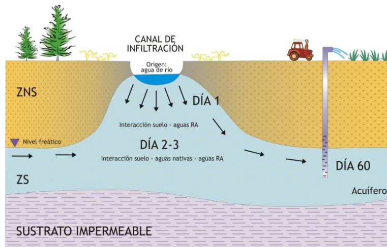
Figura 1. Esquema operativo de un dispositivo de recarga artificial de acuíferos (canal) en una zona regable.
