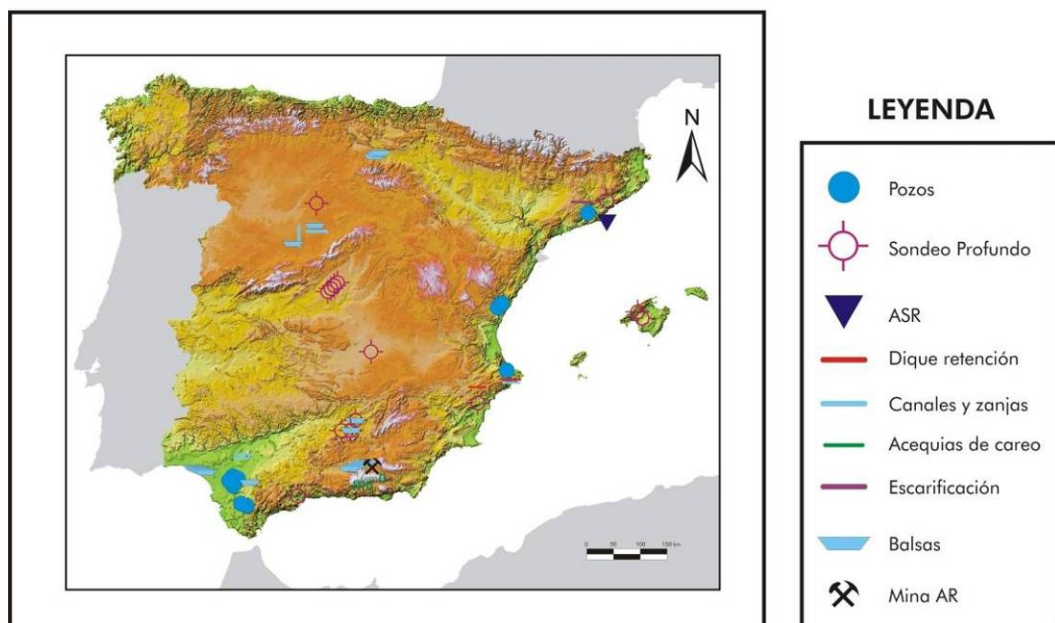
Figura 2. Principales estructuras y dispositivos de MAR operativos en España y tipologías.
